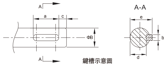
鍵槽示意圖
