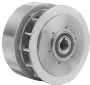
PHC 型(空心軸型)磁粉式離合器
