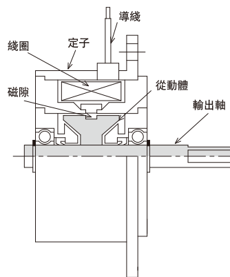
PXB 型磁粉制動器 (示意圖)
